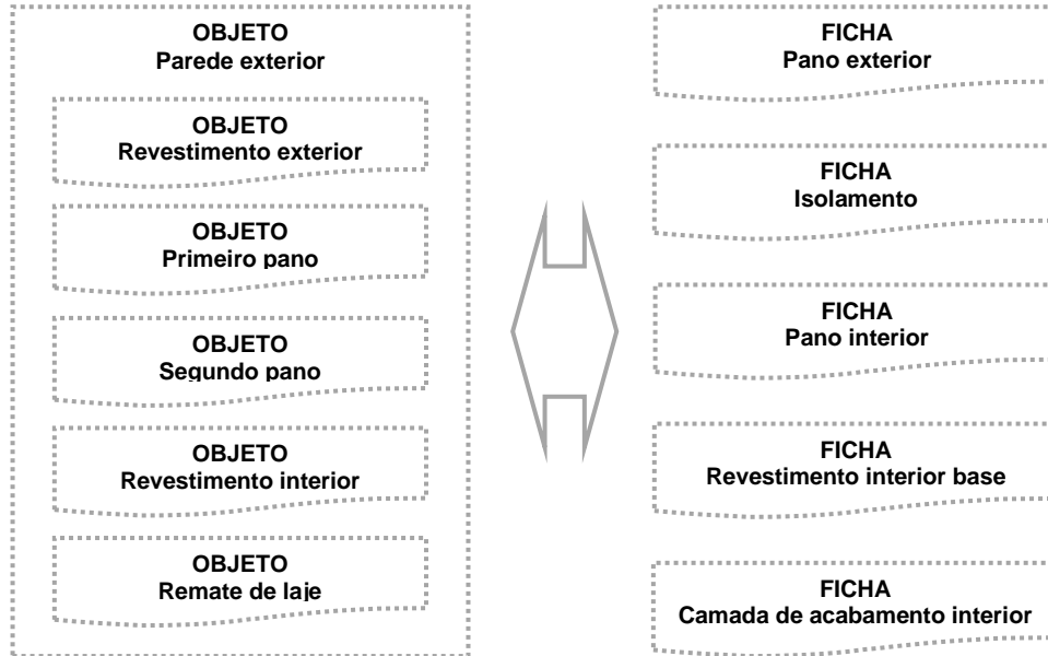
Fig.3 – Características e relação entre um objeto parede e respetivas fichas
