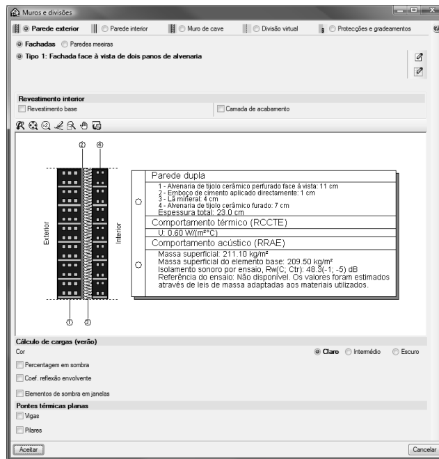
Fig.4 – Modelação de uma parede exterior no programa Instalações do edifício
