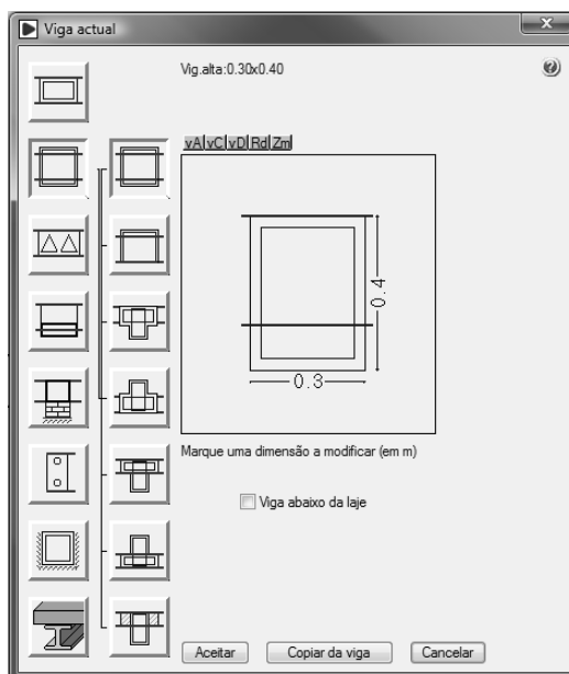
Fig.2 – Modelação de uma viga de betão armado no programa CYPECAD
